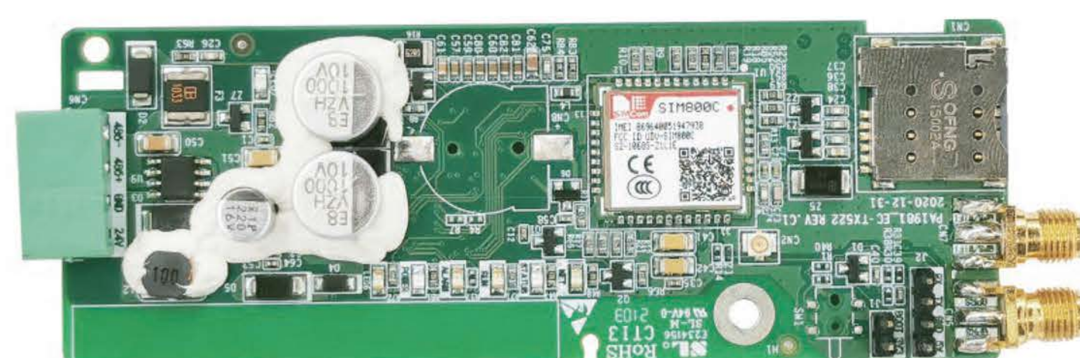
GPRS module
